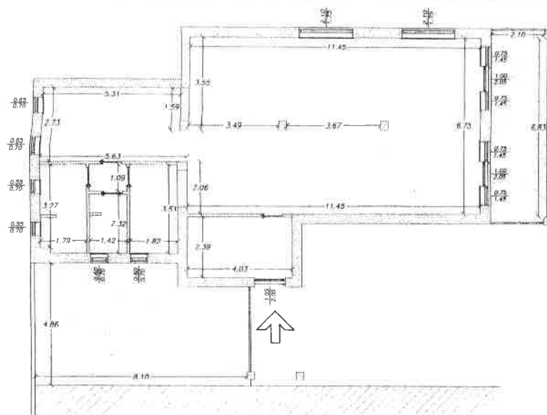
PIANTA PIANO TERRA - ASILO NIDO
